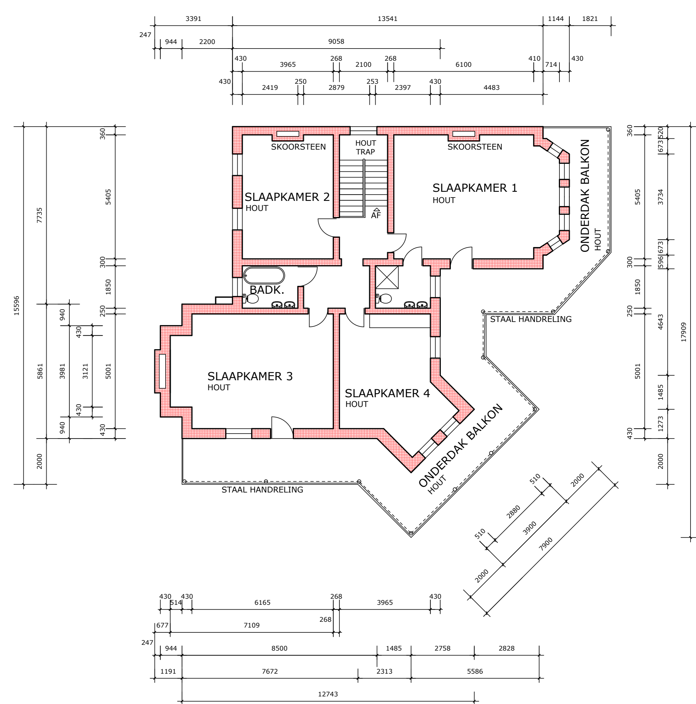
EERSTEVLOER - BESTAANDE UITLEG SKAAL 1:100 OP A0 VEL
