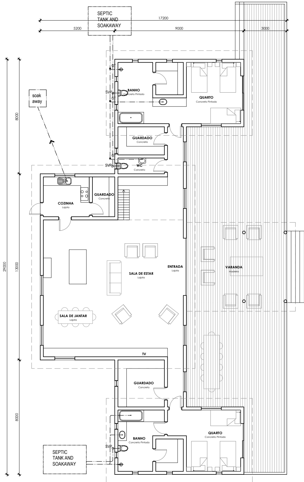
PLANO de ANDAR da TERRA-EDIFÍCIO ALOJAMENTO ESCALA 1:100
